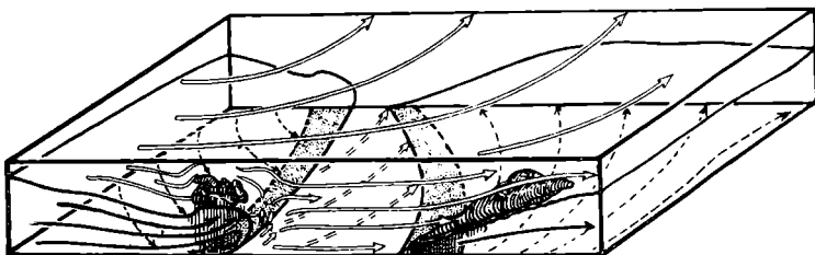
Fig. 2. Aerotektonische Skizze.
